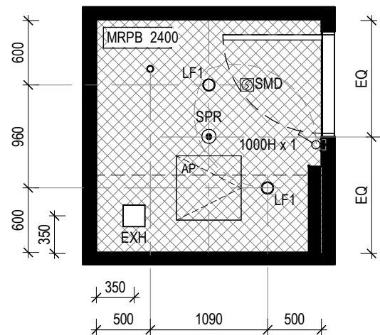
2 RCP-STANDARD ENSUITE Scale 1 : 50
