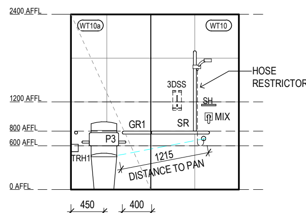
RACF - ACCESSIBLE ENSUITE ELEVATION 4 Scale 1 : 50
