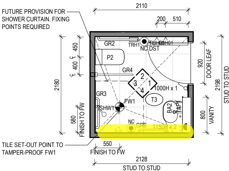
1 RACF STANDARD ENSUITE Scale 1 : 50
